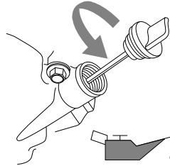
Figure 2-11. Retrait de la jauge
